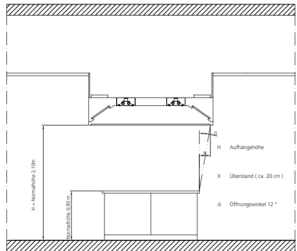
Haubenüberstand bei höherer Aufhängung
